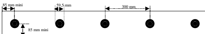
FIGURE 8: CIBLERIE VITESSE 5 CIBLES
