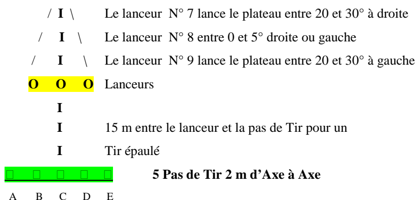
FIGURE 16: PAS DE TIR « CADETS » SUR FOSSE OLYMPIQUE
